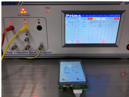
图 6-3 群脉冲测试图
