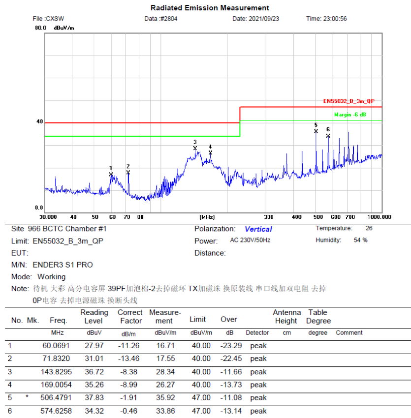
图 6-6 辐射测试垂直方向
