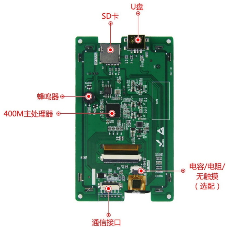
图 1-4 硬件配置图
