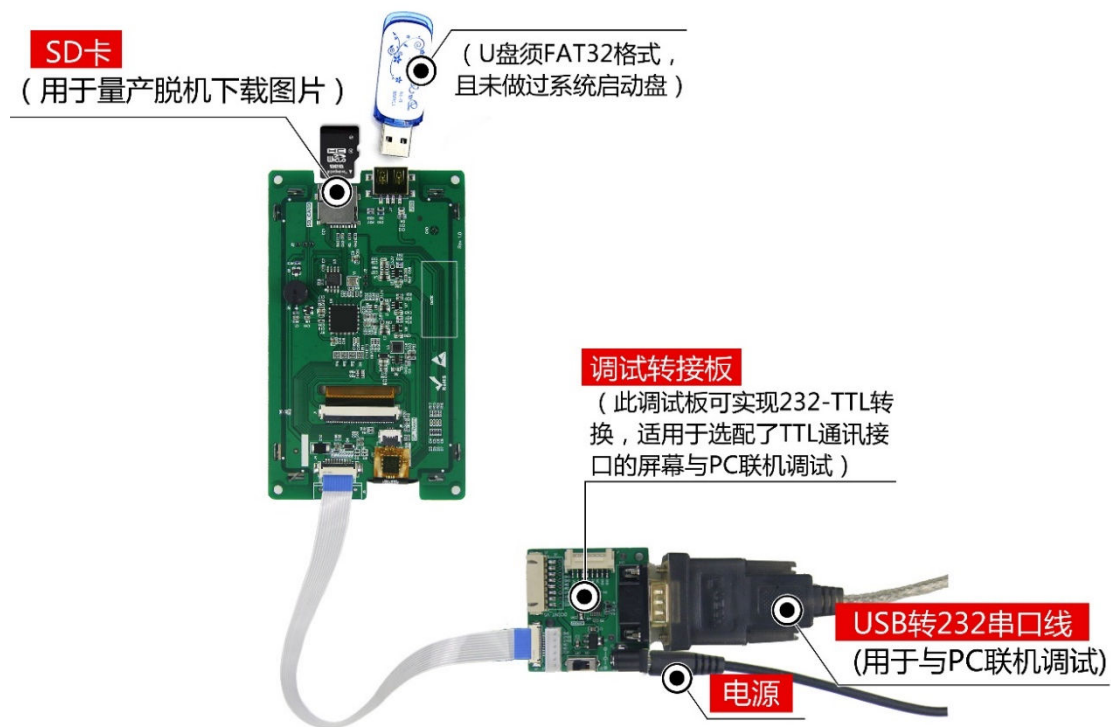
图 1-5 调试工具图
