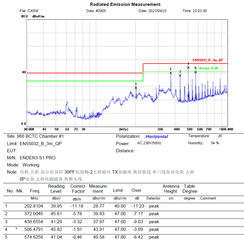
图 6-5 辐射测试水平方向
